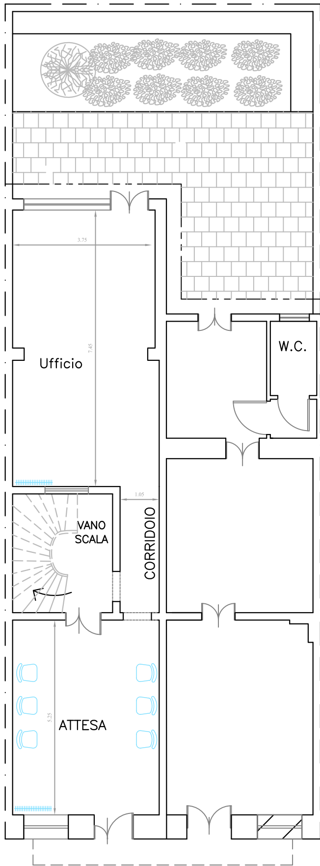
PIANTA ARREDATA PIANO TERRA Via Granafei 53 - Mesagne
